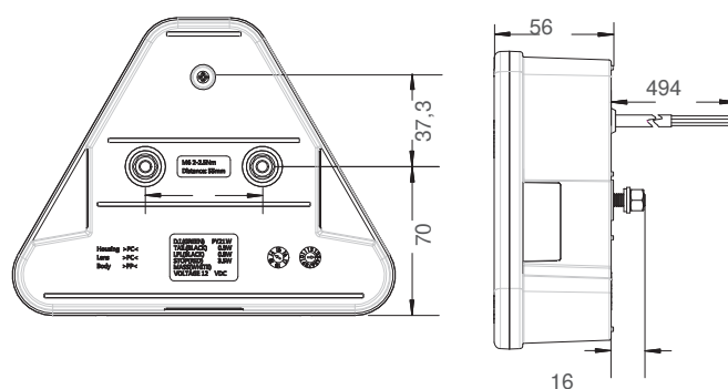
0,5 M KABEL MIT OFFENEM ENDE 0.5 M OPEN ENDED CABLE
