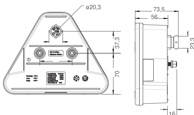
5 POL. BAJONETTANSCHLUSS 5 PIN BAYONET CONNECTOR
