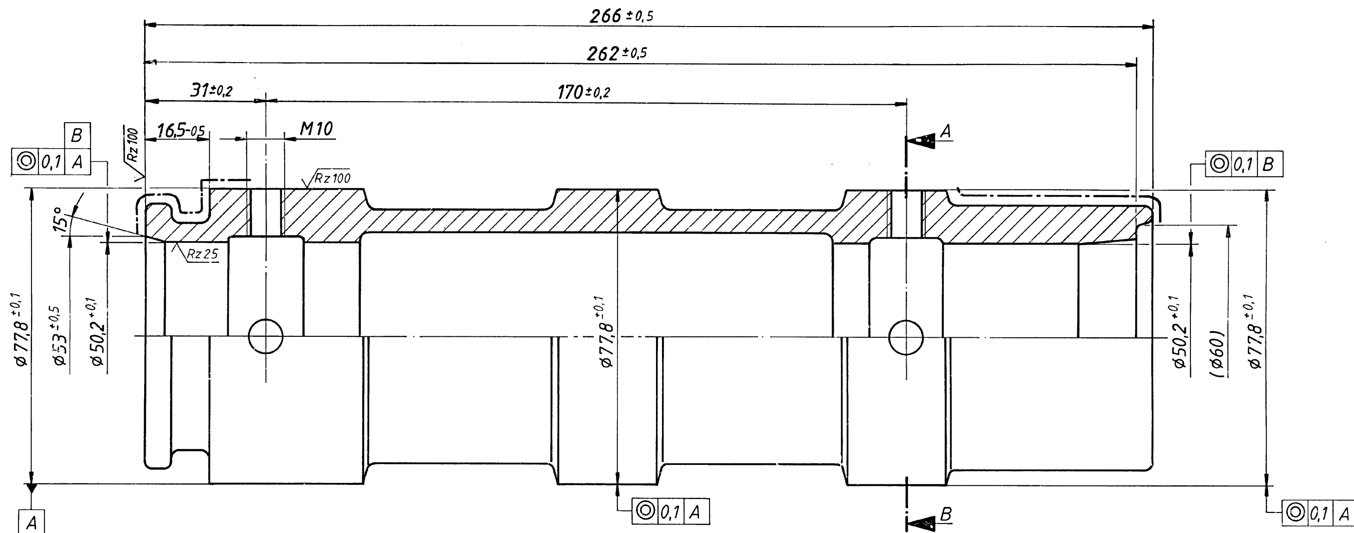
Schnitt A-B
