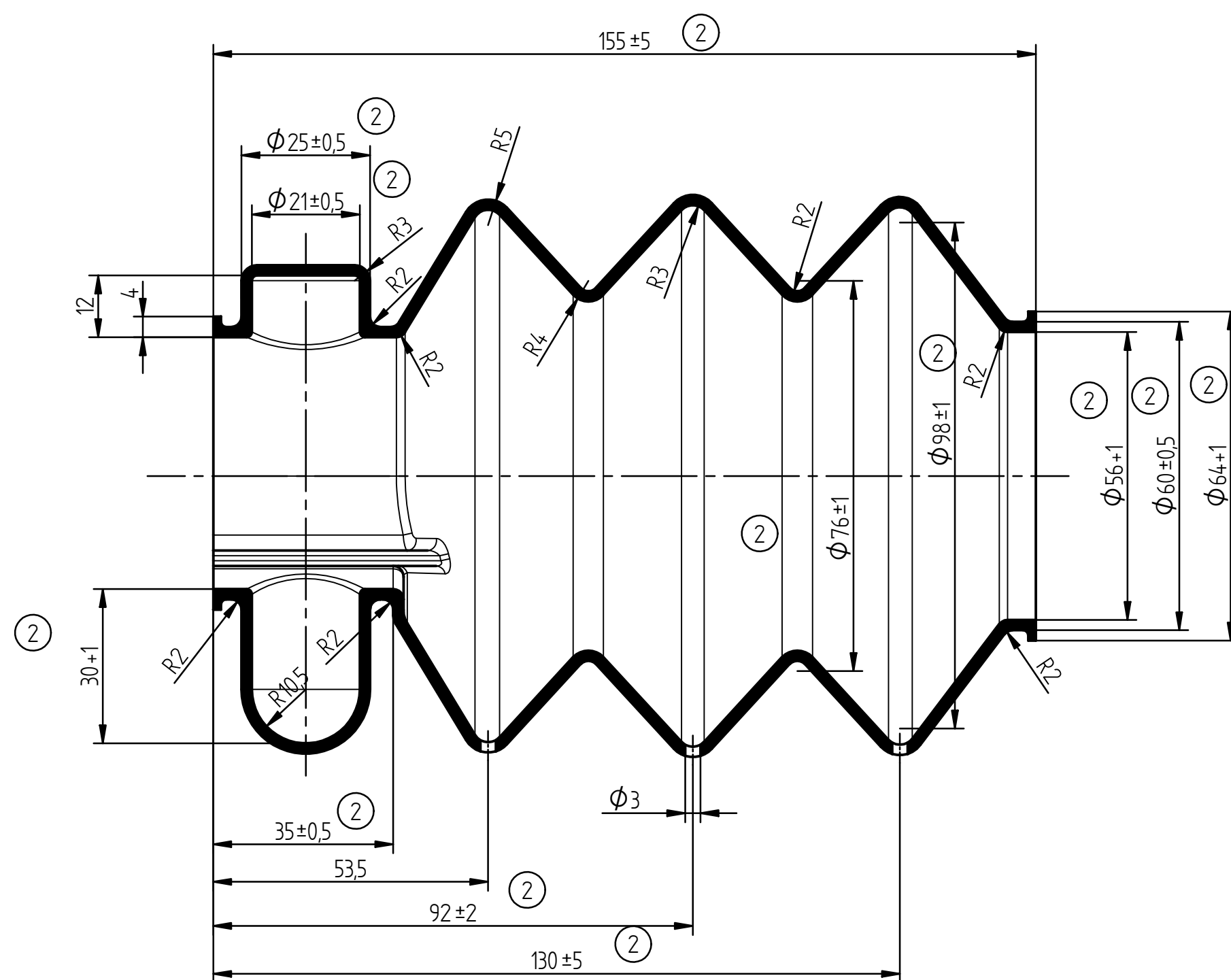
Schnitt A-A
